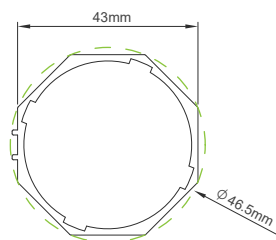
ATO43 八角管 #09602E05X
