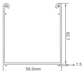
62 軌道 #09603I092(白色) #09603I091(核桃木色)
